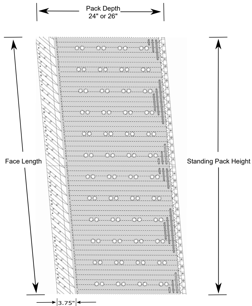
XF 75 IL Side View
